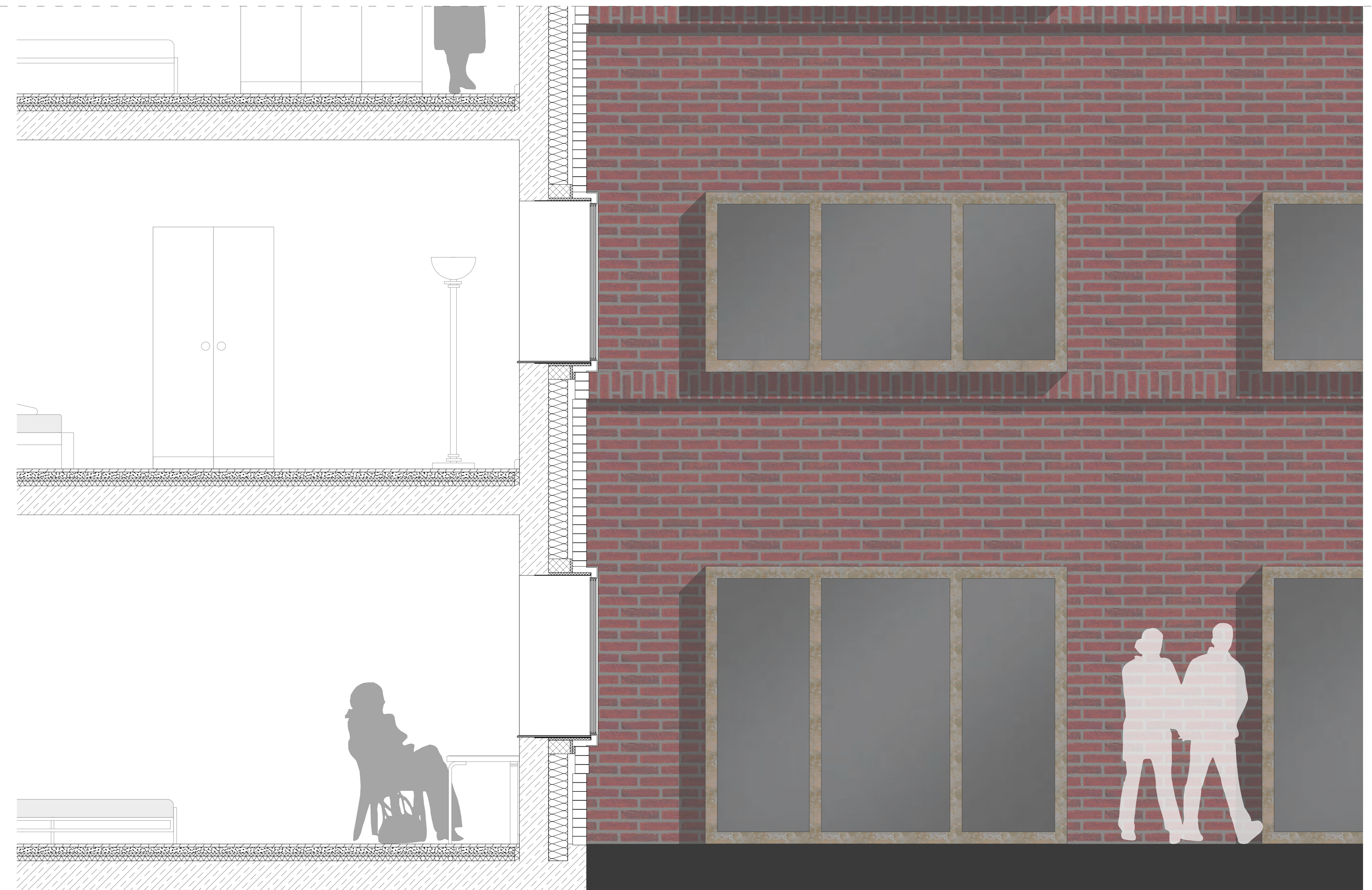
Fassadenschnitt 1:20
