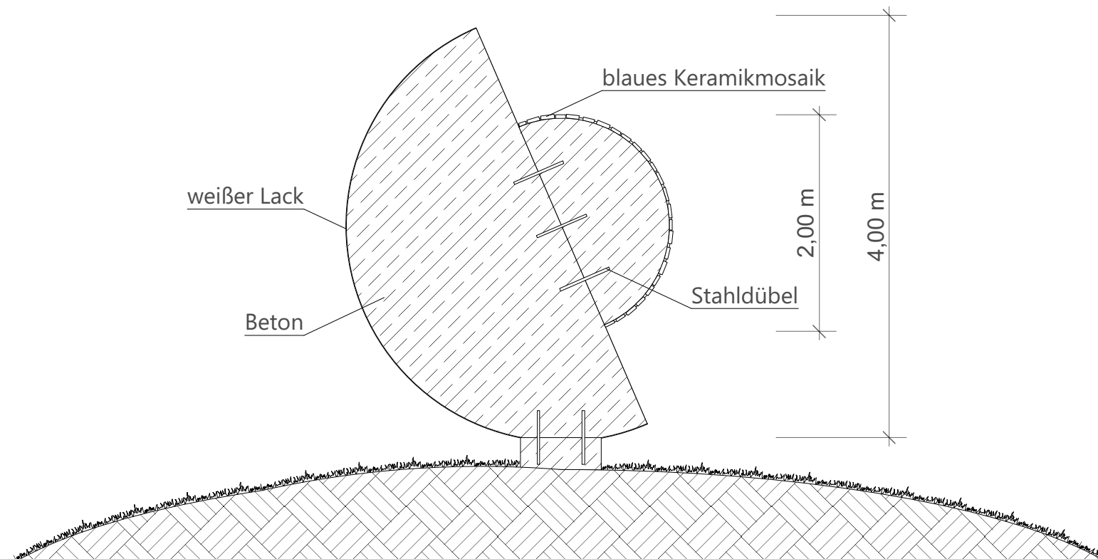
Konstruktionsschnitt Maßstab 1:50
