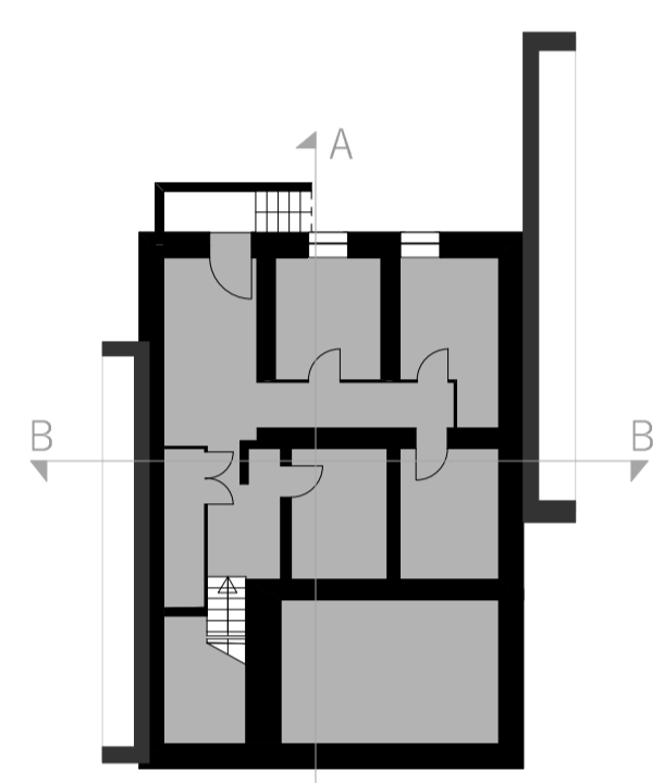
KG Bestand | 1:200
