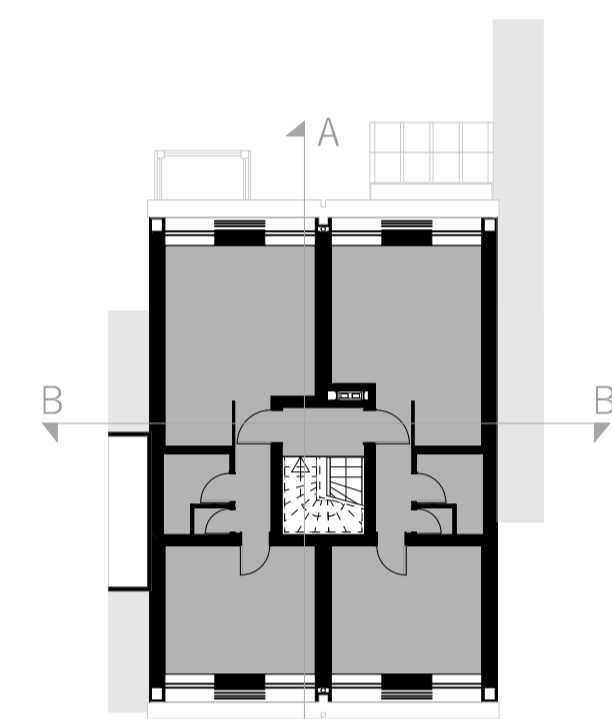
DG 2 Erweiterung | 1:200
