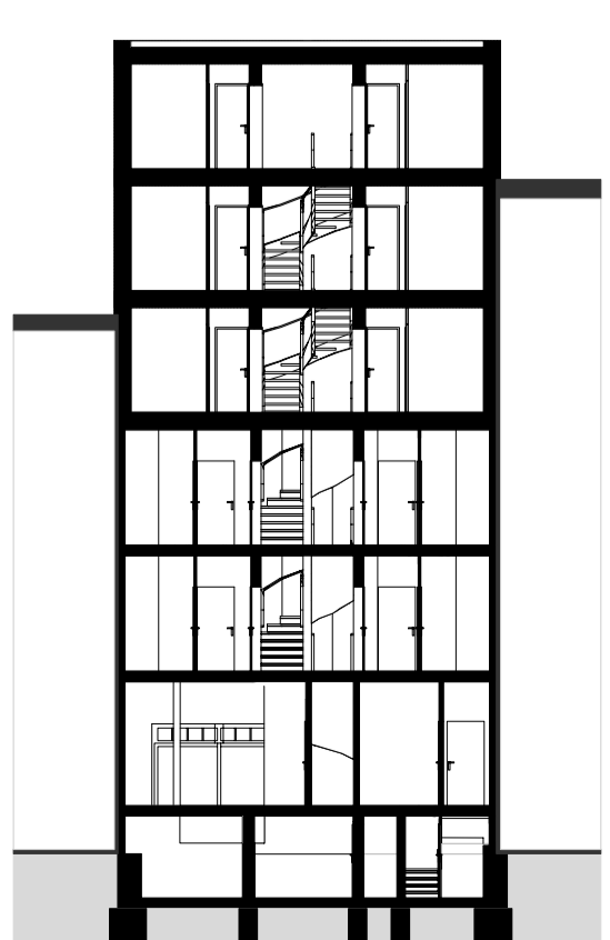
Schnitt AA | 1:200
