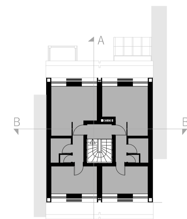
DG 3 Erweiterung | 1:200
