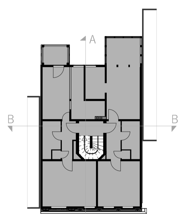
1. OG Bestand | 1:200
