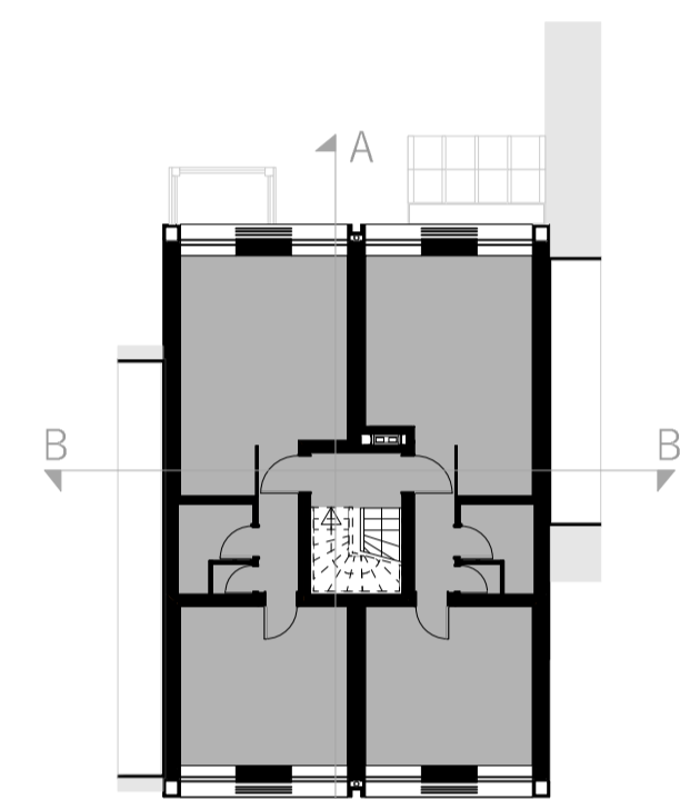
DG 1 Erweiterung | 1:200
