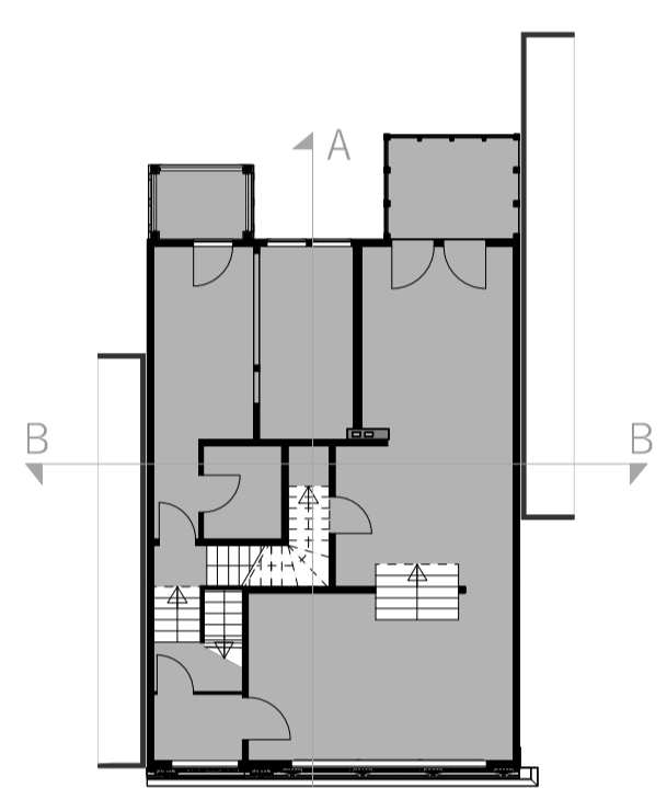
EG Bestand | 1:200
