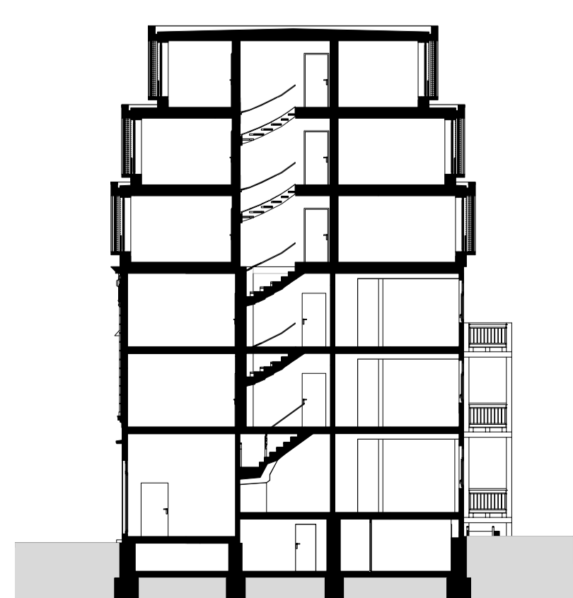
Schnitt AA | 1:200
